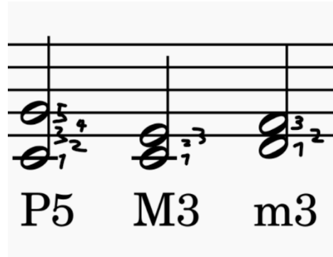
図 11: 音程
